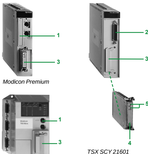
TSX SCY 21601
