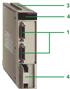
TSX CTY 2C
